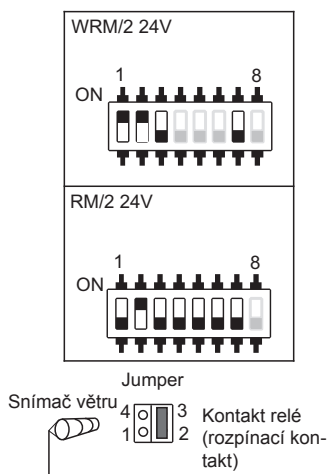
Nastavení spínače DIP
