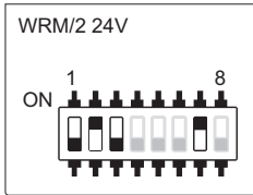
DIP-Schaltereinstellung
